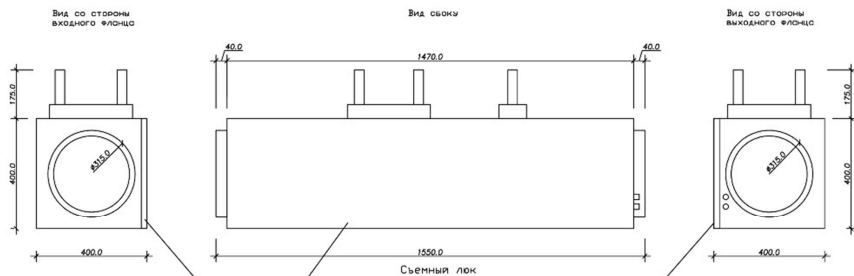
Габаритные и присоединительные размеры. Варианты исполнения.
