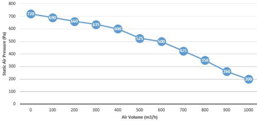
Приточная установка Aiken EV-1000
